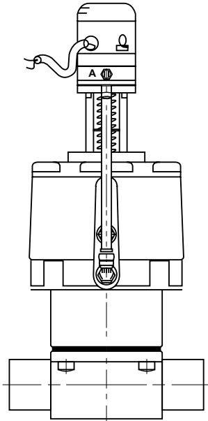
Mini electropneumatic positioner mounted on an EC actuator
